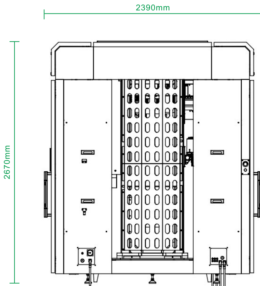
前视图
